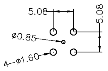
PCB LAYOUT(REF)
